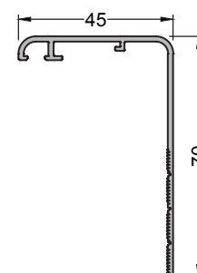
801-070 ( 0,525 kg/mt ) AW13 SILL PROFILE
